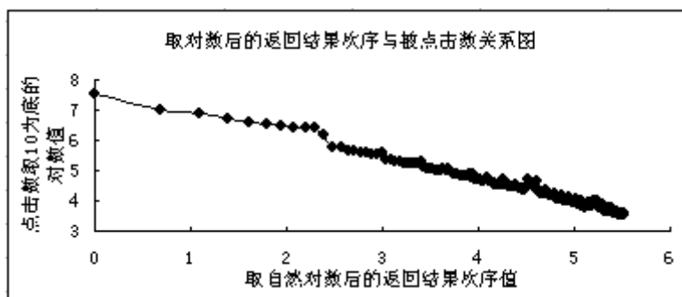
图 4 对返回结果的顺序排名与被点击次数取对数值后的关系
