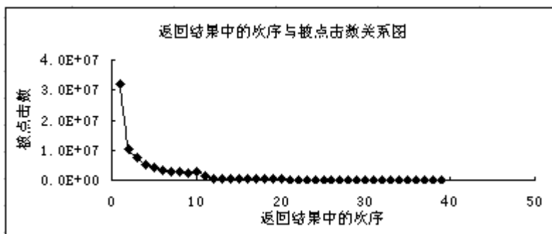
图 3 返回结果的顺序排名与被点击次数的关系
